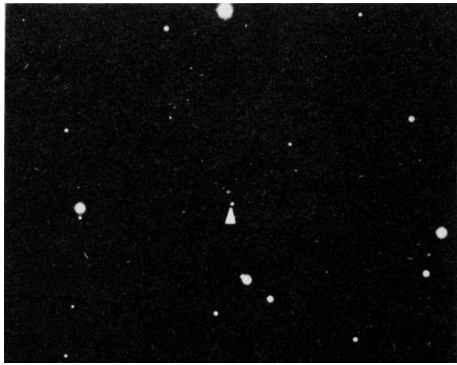
图 5.7: 和我们银河系一样的一个螺旋银 图 5.8: 最现代化的 200 英寸望远镜拍摄 河系，假定它的直径与我们银河系相近，那 的最远天体——牧夫座中的 3C295（用箭 么我们从它的表观大小就能算出它的距离。头标出） 它离地球约 3000 万光年（即 3 \times 10^{23} 米）
