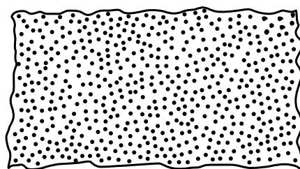
图 5.10: 在只观察核的时候，通过一块厚 1 厘米的碳所见到的那个设想的图像
